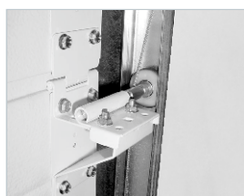
Charnières latérales avec support roulette (laquées blanches)
