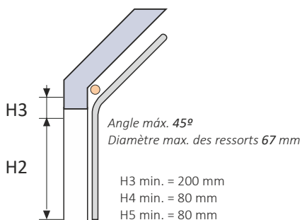
INCLINÉ RES200i
