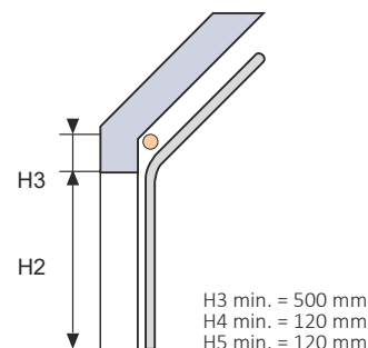
INCLINÉ IND-IL
