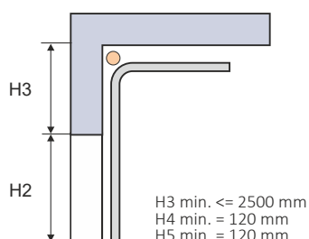
HAUT IND-HL1
