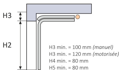
RÉDUIT RES100
