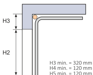
RÉDUIT IND-RL
